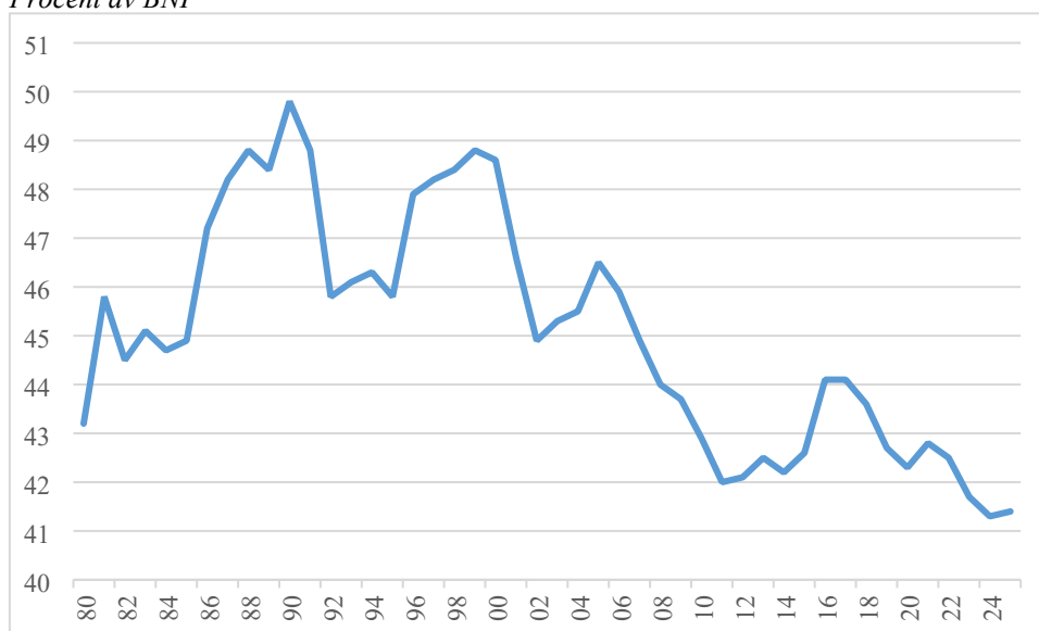
Figur 22 Skattekvoten 1980–2025
