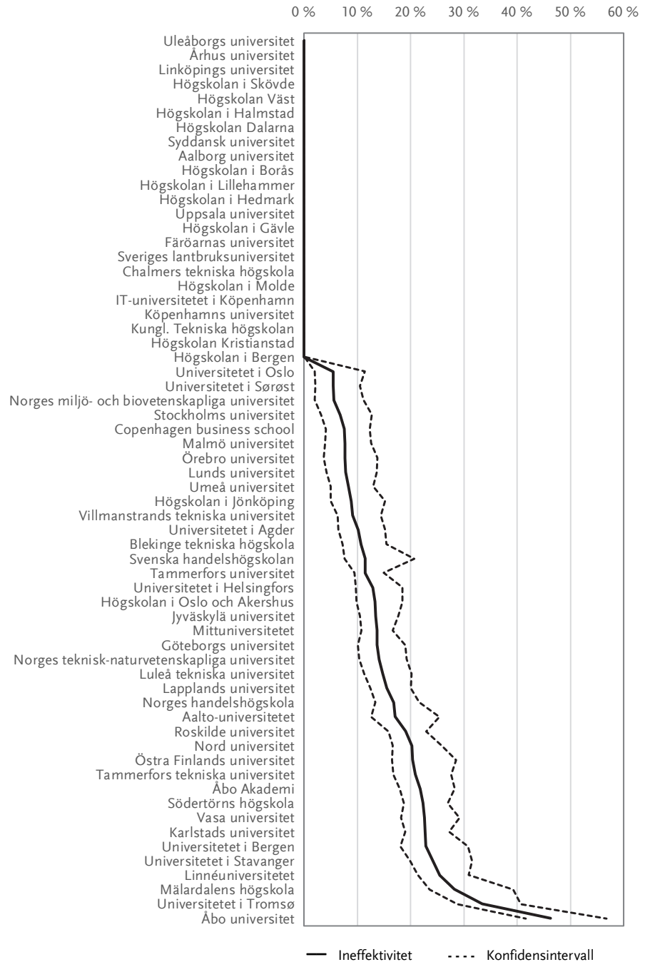
Diagram B5 Ineffektivitet för nordiska lärosäten år 2015, konstant skalavkastning med konfidsensintervall
