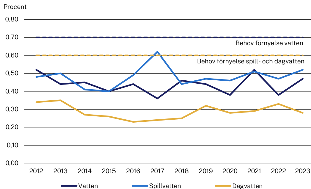
Diagram 1. Faktisk förnyelse och behovet enligt Svenskt Vatten uppskattade behovet av förnyelse av ledningsnät, uppdelat på vatten samt spill- och dagvatten, 2012–2023
